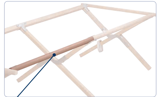
Längsstrebe Nr. 93-5995
